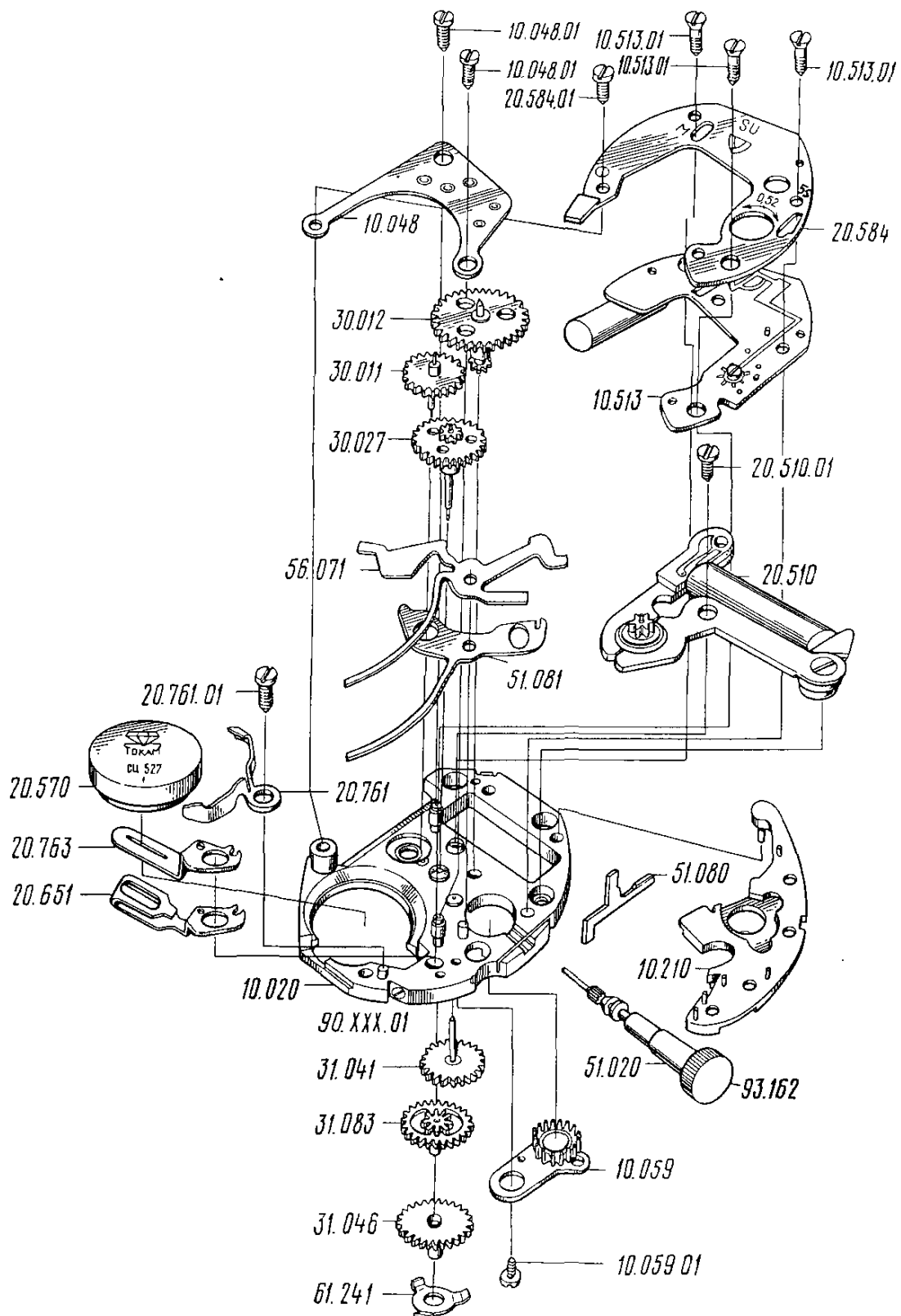
Рис. 19. Детали и сборочные единицы механизма часов 1356:
