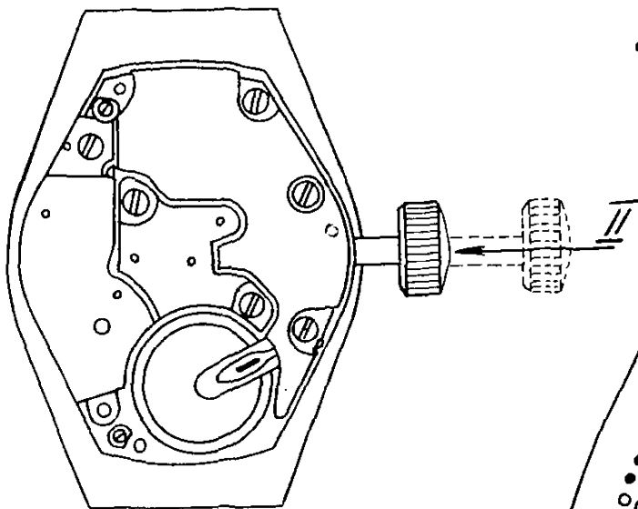
Рис. 94. Извлечение механизма из корпуса: I – для извлечения механизма из корпуса необходимо вынуть из механизма вал переводной, нажав на ось рычага переводного концом линцета или отвертки; II – установить вал переводной в механизм
