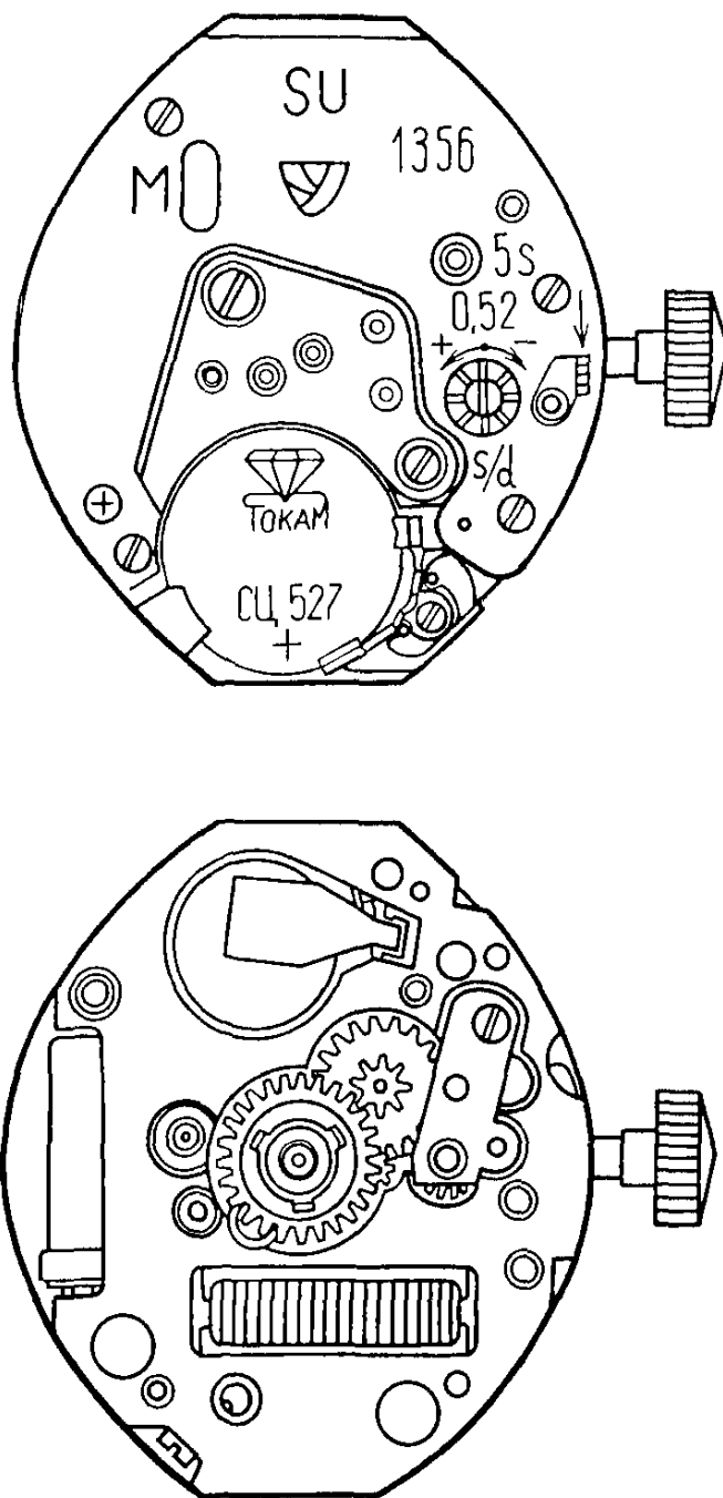
Рис. 18. Механизм часов 1356
