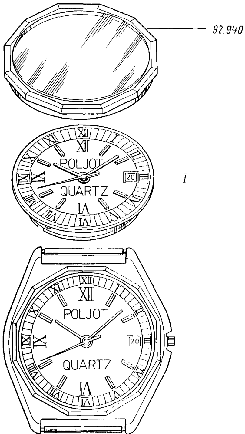
Рис. 158 92.940 – ободок; i – для извлечения механизма из корпуса необходимо снять ободок со стеклом
