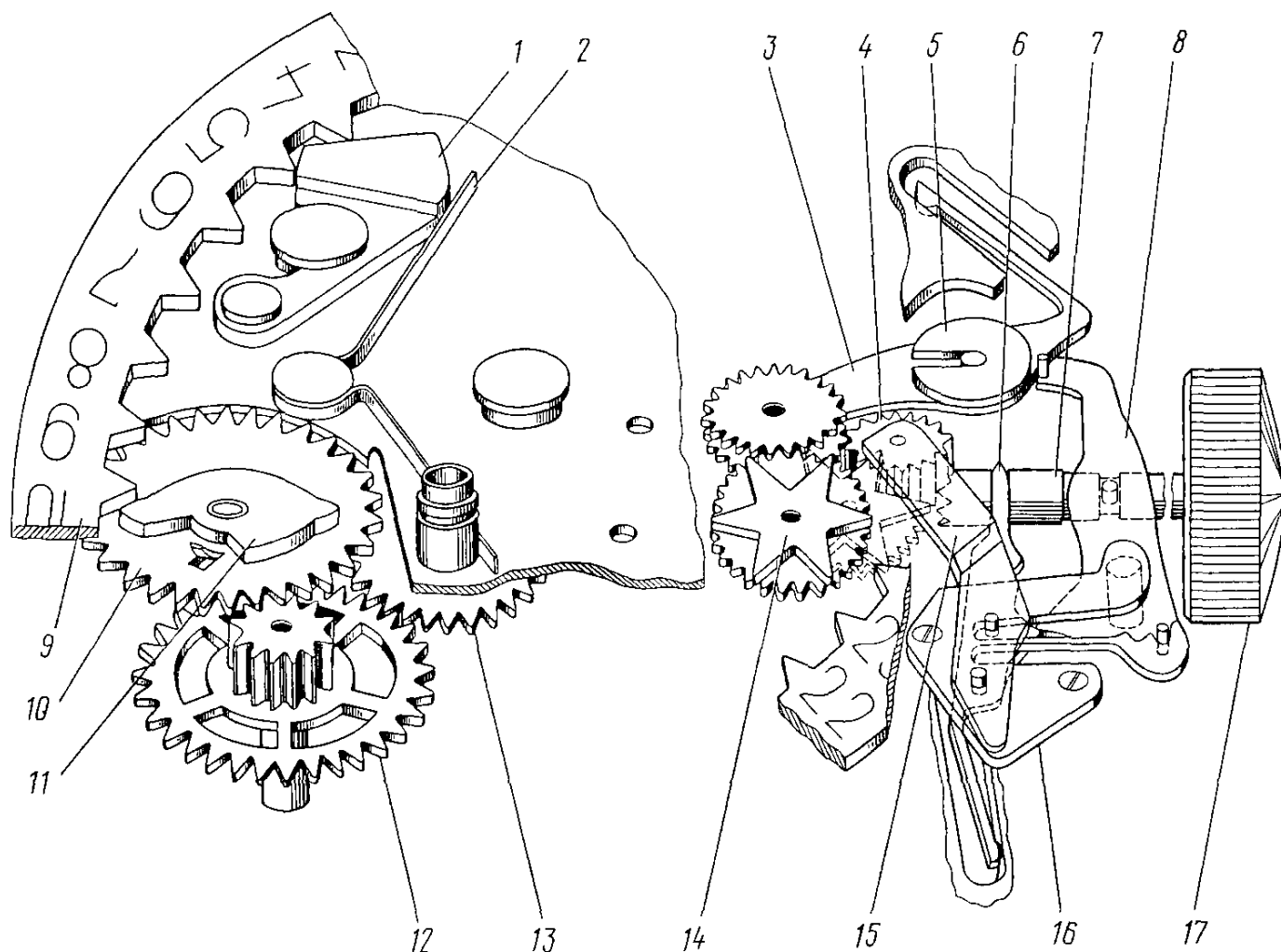
Рис. 8. Кинематическая схема календарного устройства механизма часов 2460:
