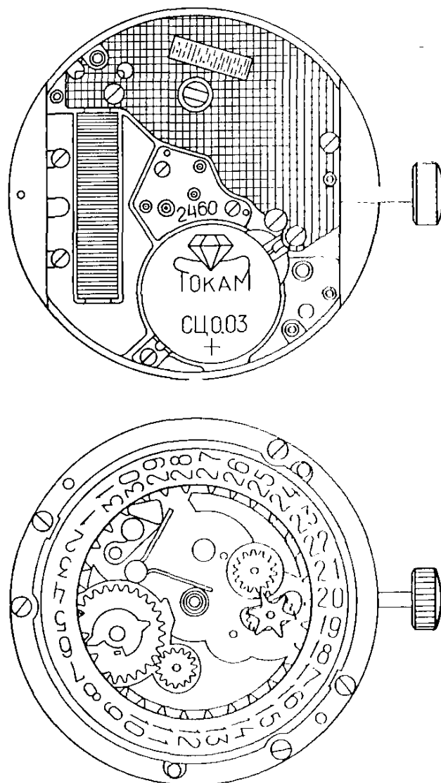
Рис. 156. Механизм часов 2460
