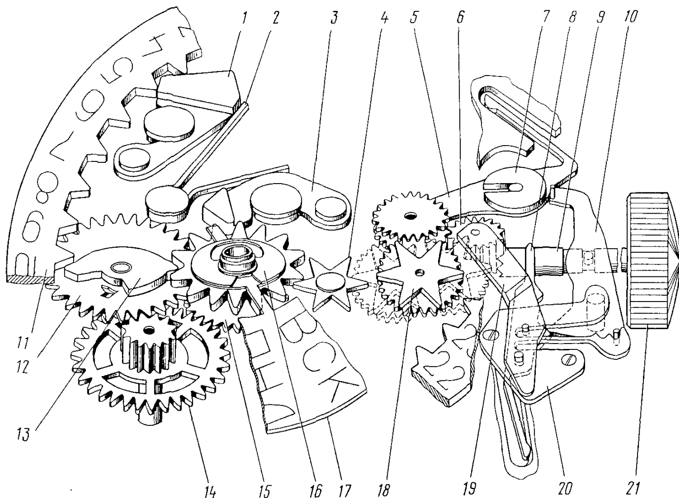
Рис. 7. Кинематическая схема календарного устройства механизма часов 2450:
