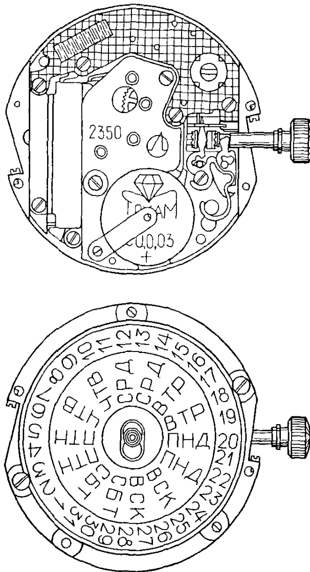
Рис. 112. Механизм часов 2350
