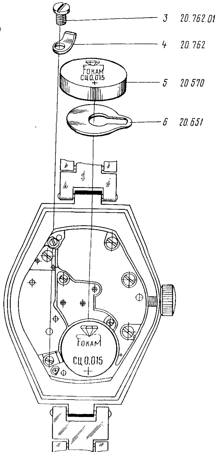
Рис. 93 Примечание: источник питания брать только пластмассовым пинцетом или пинцетом с изолированными концами.
