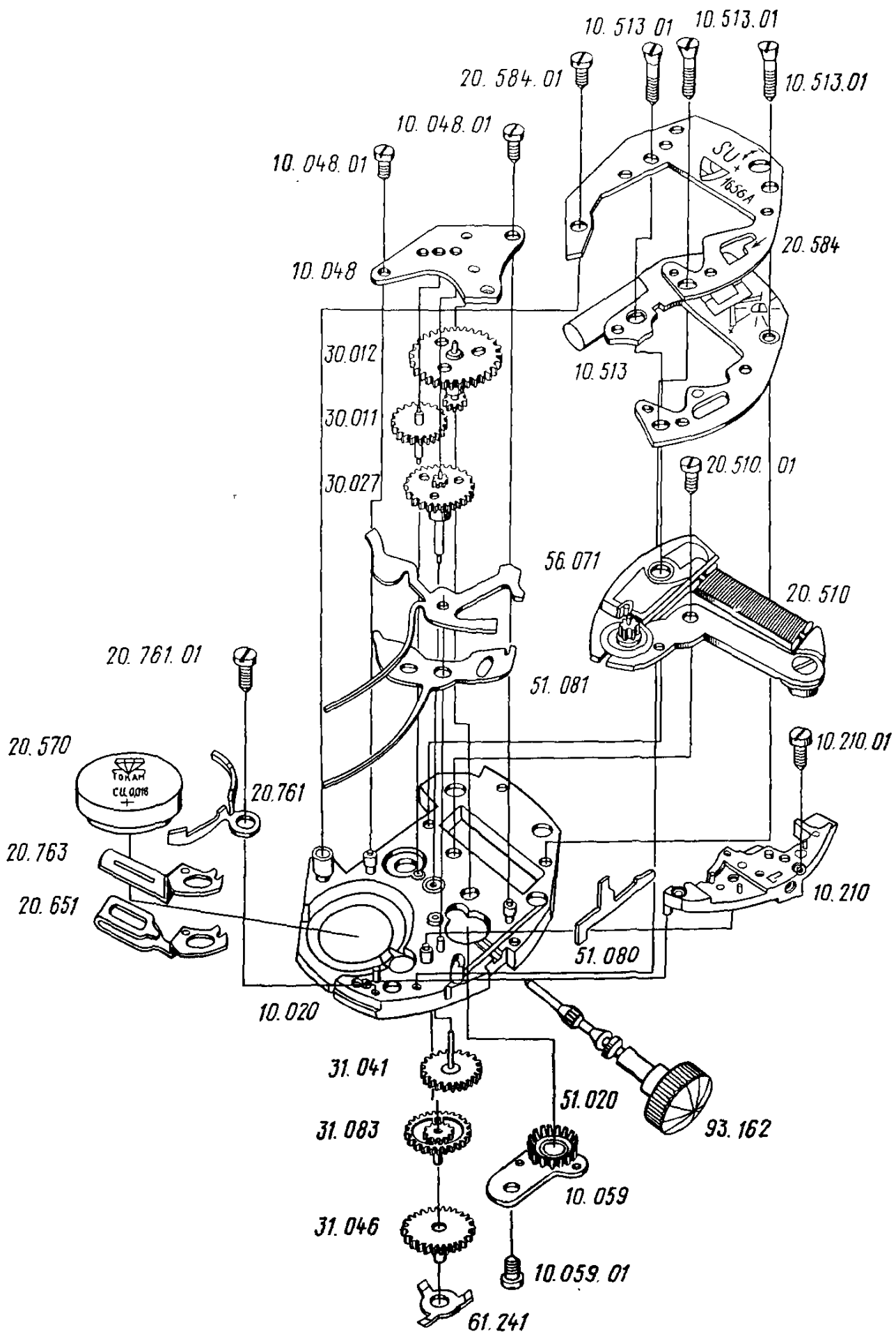
Рис. 65. Детали и сборочные единицы механизма 1656А:
