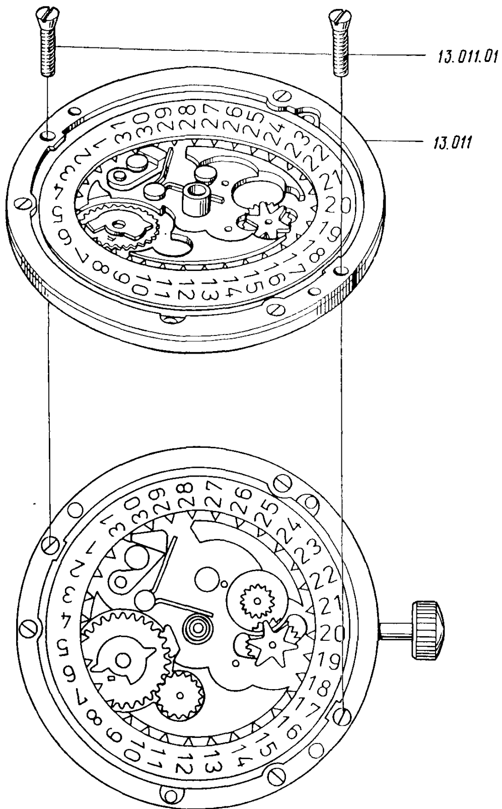
Рис. 160 13.011 – блок календаря; 13.011.01 – винт блока календаря.
