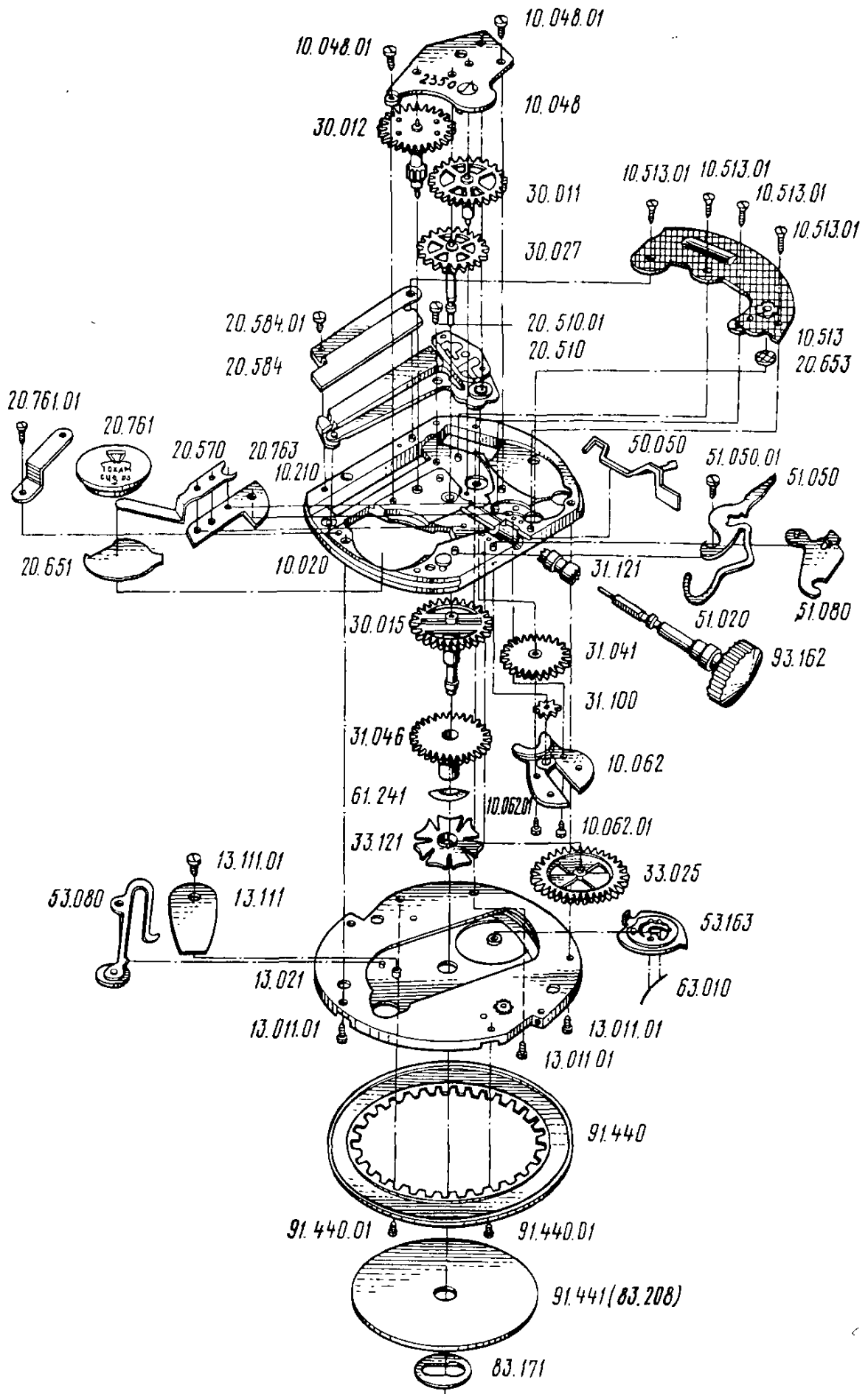
Рис. 113. Детали и сборочные единицы механизма часов 2350, 2360: 10.020 – плата; 10.048 – мост колесной передачи; 10.048.01 – винт моста колесной передачи; 10.062 – мост колеса минутного; 10.062.01 – винт моста колеса минутного; 10.210 – накладка; 10.513 – блок кварцевого генератора; 10.513.01 – винт блока кварцевого генератора; 13.011.01 – винт блока календаря; 13.021 – плата календаря; 13.111 – пластина фиксатора чисел месяца; 13.111.01 – винт пла-
