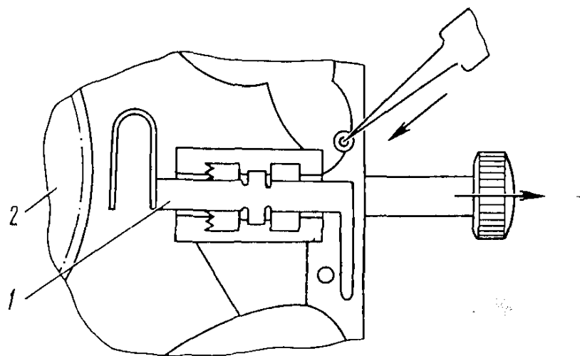
Рис. 14. Извлечение вала переводного из механизма КНЧ 1656Н: 1 – тормозной рычаг; 2 – колесо секундное
