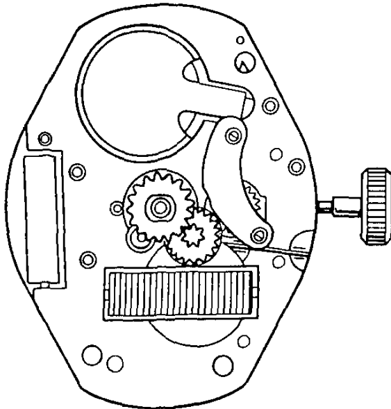
Рис. 44. Механизм часов 1656
