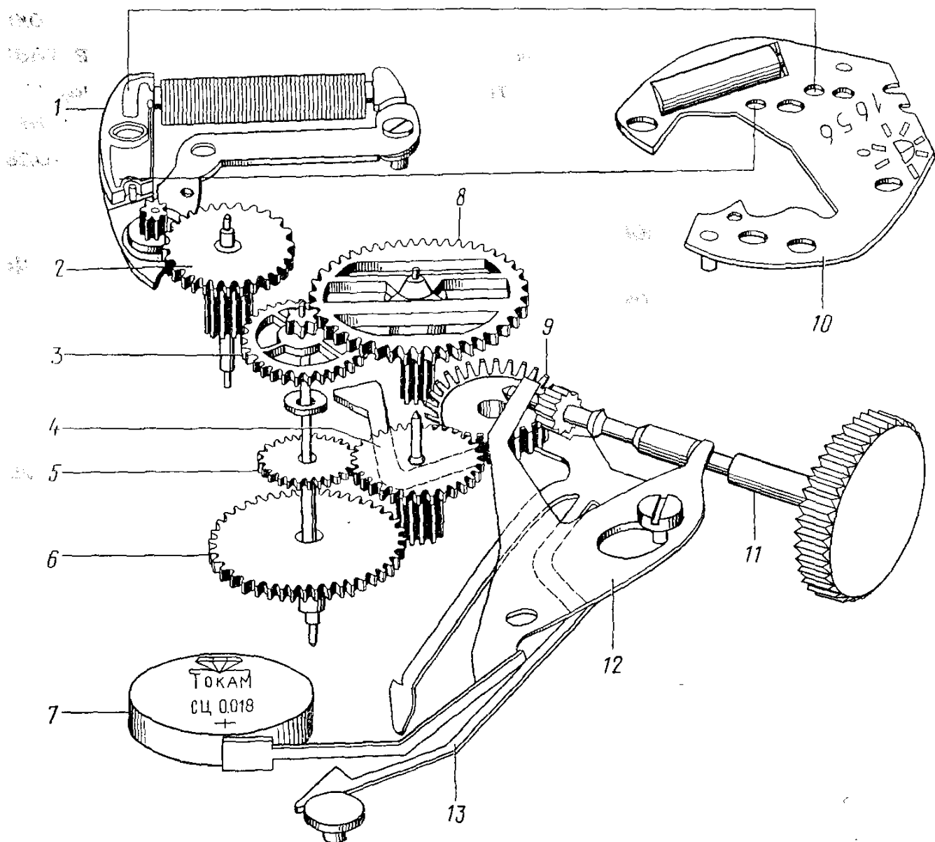
Рис. 3. Кинематическая схема механизма часов 1656: 1 – шаговый двигатель; 2 – колесо передаточное; 3 – колесо секундное; 4 – колесо минутное; 5 – триб минутный свободный; 6 – колесо часовое; 7 – источник питания; 8 – колесо промежуточное; 9 – колесо переводное; 10 – блок кварцевого генератора; 11 – вал переводной; 12 – токосъемник боковой; 13 – стопор промежуточного колеса
