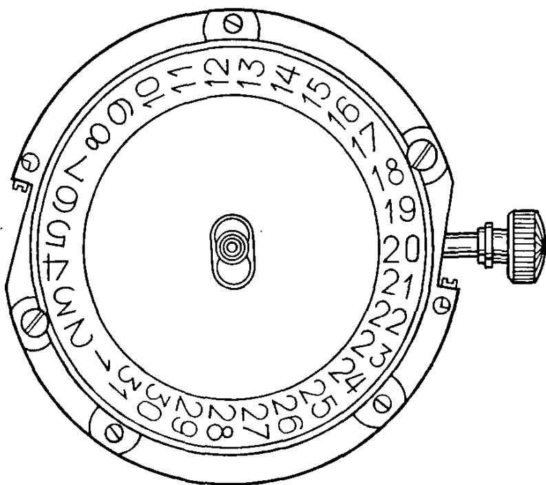
Рис. 133. Механизм часов 2360
