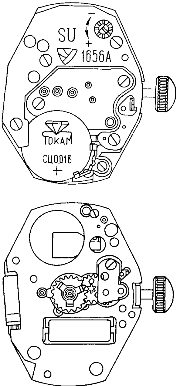
Рис. 64. Механизм часов 1656А
