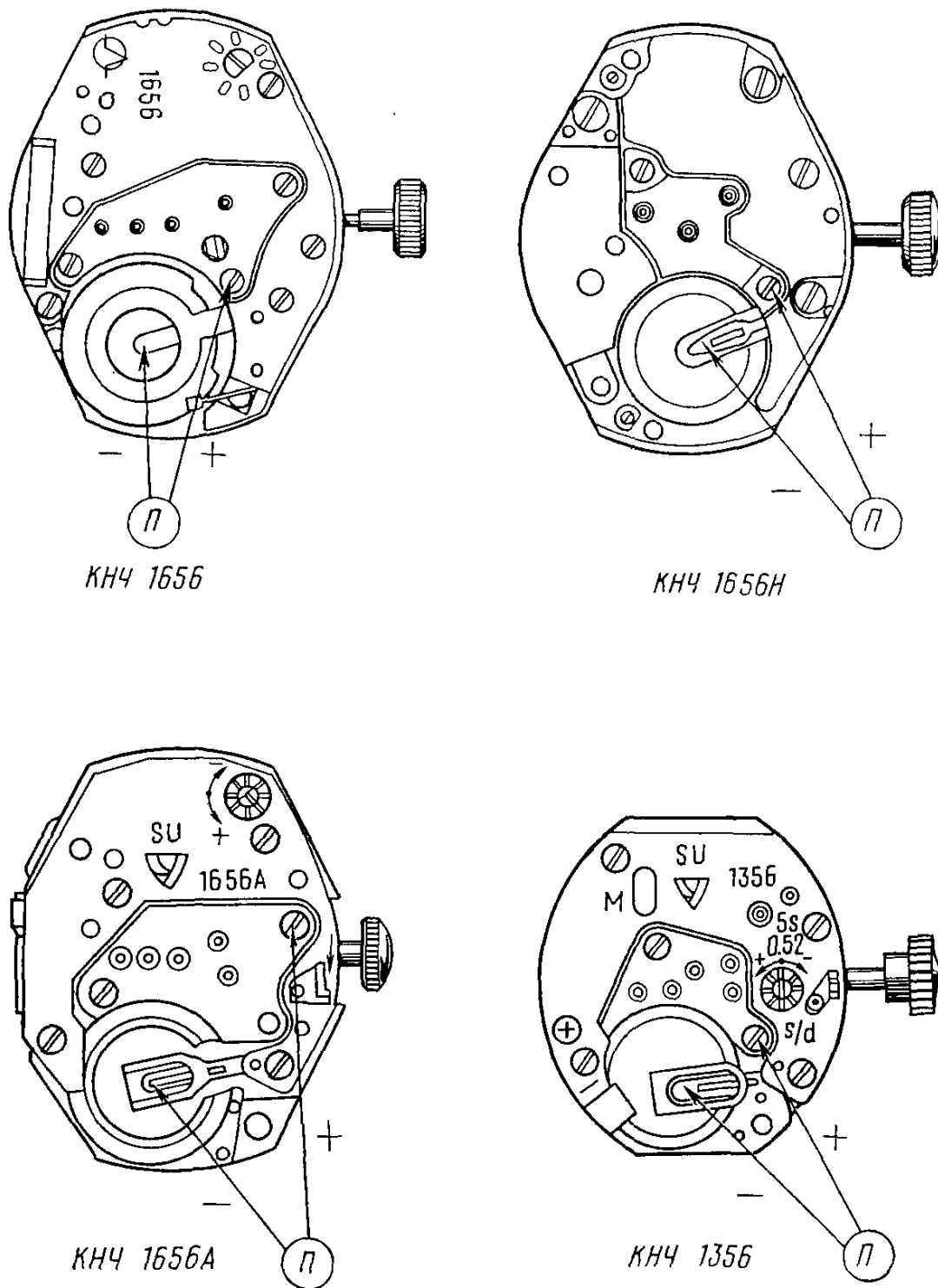
Рис. 17. Установка щупов прибора П157А для измерения тока, потребляемого часами: П – прибор П157А
