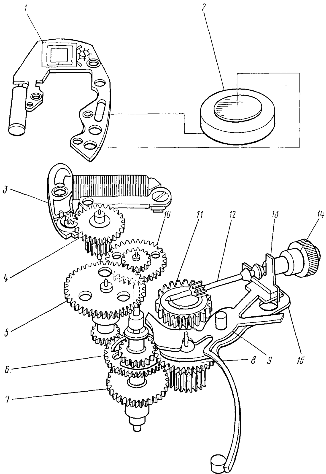
Рис. 4. Кинематическая схема механизма часов 1656А: 1 – блок кварцевого генератора; 2 – источник питания; 3 – шаговый двигатель; 4 – колесо передаточное; 5 – колесо промежуточное; 6 – колесо центральное; 7 – колесо часовое; 8 – колесо минутное; 9 – рычаг обнуления; 10 – колесо секундное; 11 – колесо переводное; 12 – вал переводной; 13 – пластина; 14 – головка переводная; 15 – рычаг переключения
