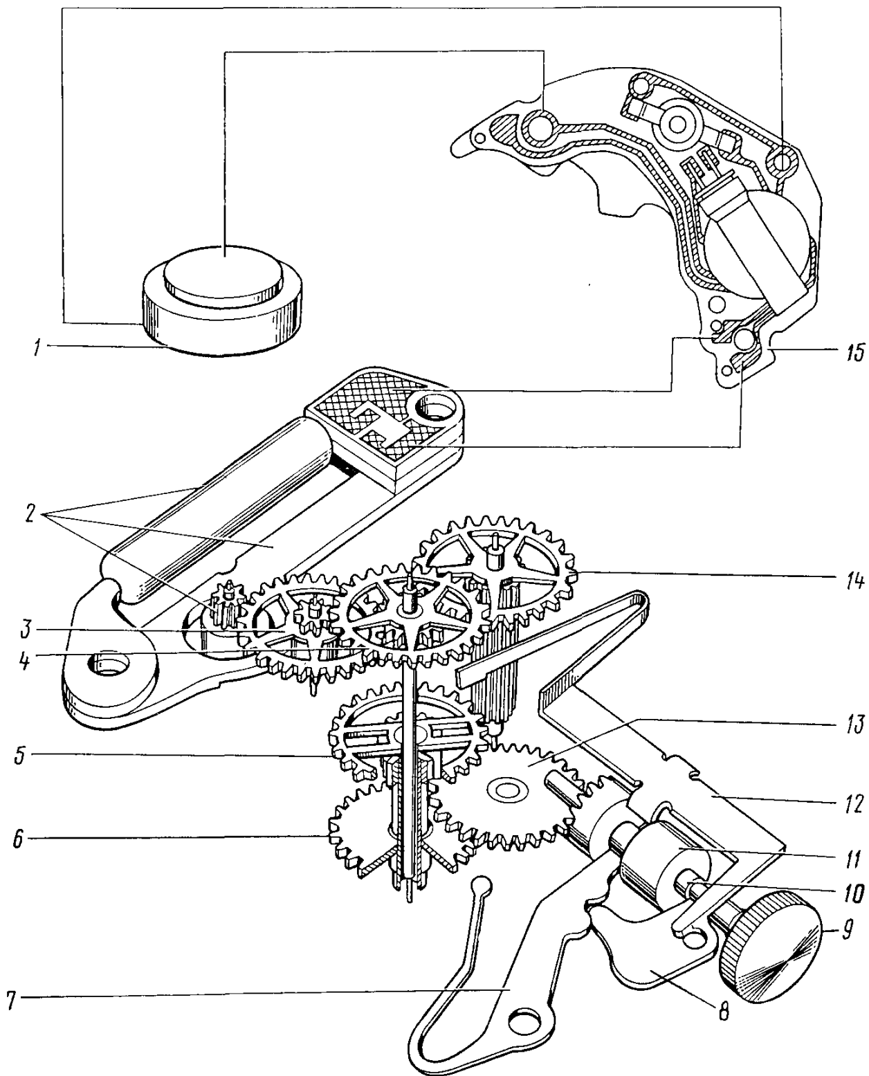
Рис. 5. Кинематическая схема механизма часов 1656H:
