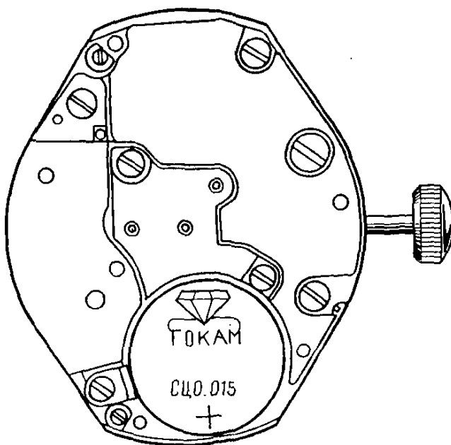
Рис. 90. Механизм часов 1656Н
