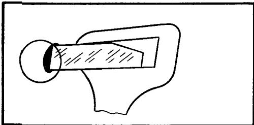
При взятии масла из масленки маслodoзиро- вку следует держать под углом 60^\circ и погружать в масленку на высоту лопаточки. Масло должно быть только на плоскостях импульса и покоя
