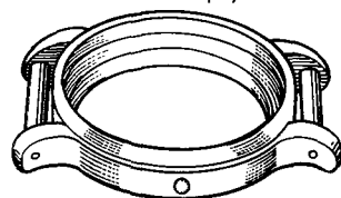
Кольцо корпусное 92.900
