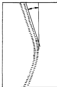
Дефект зубчатой передачи
