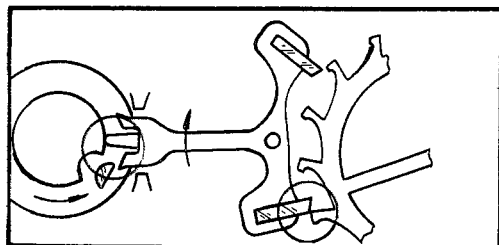
При правильном соотношении параметров хода не должно быть наскака эллипса на рожек
