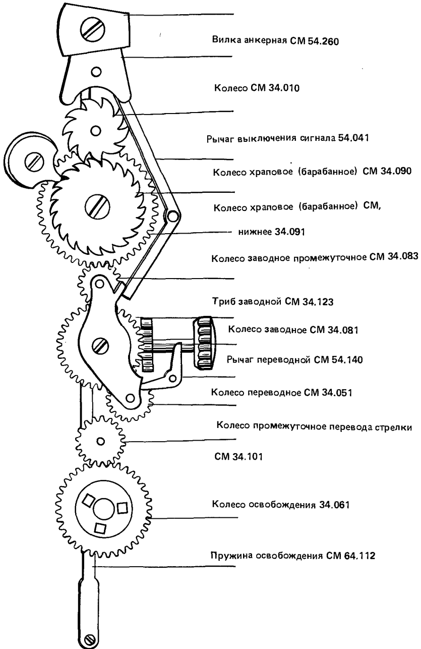
Молоточек сигнального механизма (СМ) 54.261
